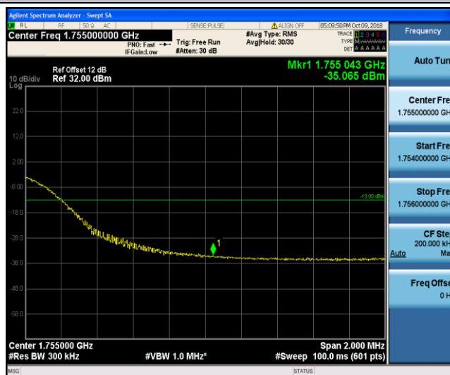
Band4 20MHz QPSK 20300 100RB#0
