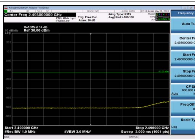
FDD07_5MHz_2502.5_Q16_OneRB_low _ExtraBands_Range_2490~2496
