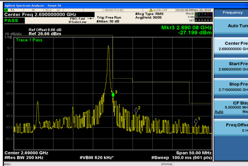
Band41-20MHz-16QAM-41490-1RB#99
