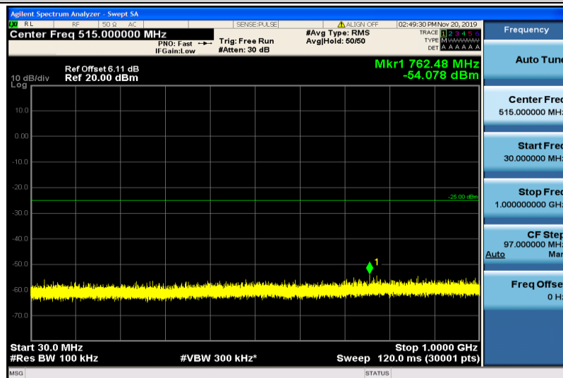
Band41-10MHz-QPSK-39700-1RB#0-30~1000MHz
