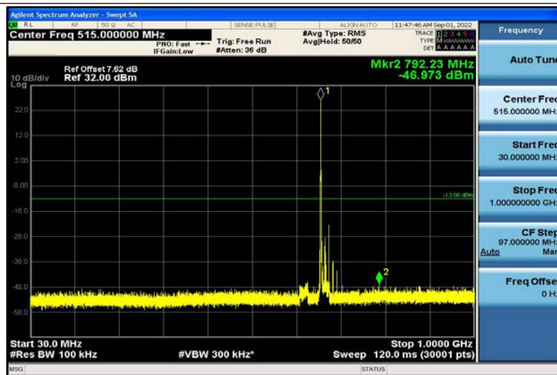
Band71-20MHz-QPSK-133222-1RB#0-30~1000MHz
