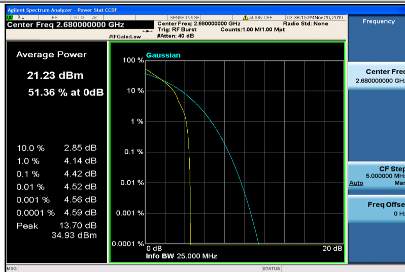
Band41-20MHz-QPSK-41490-1RB#0
