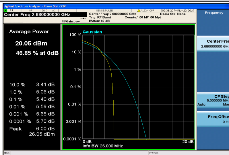
Band41-20MHz-16QAM-41490-1RB#0
