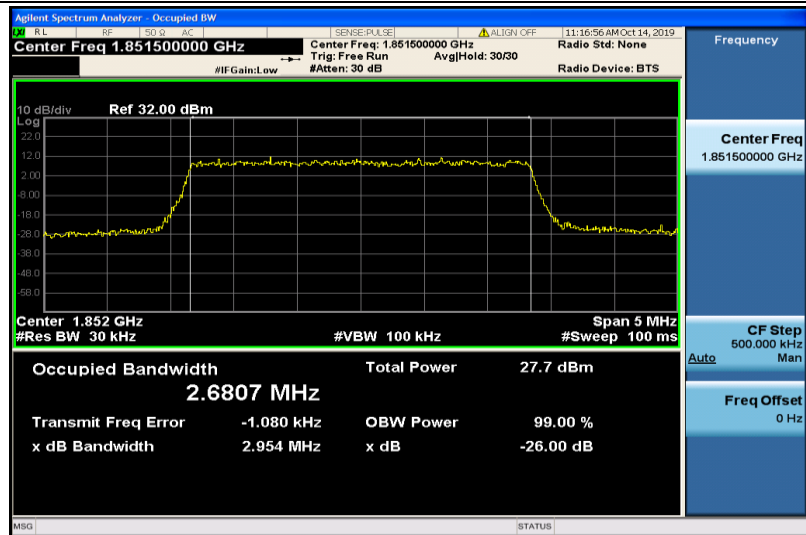
Band2-3MHz-16QAM-18615-15RB#0-2.6807
