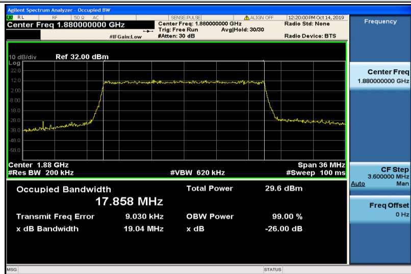
Band2-20MHz-QPSK-18900-100RB#0-17.858
