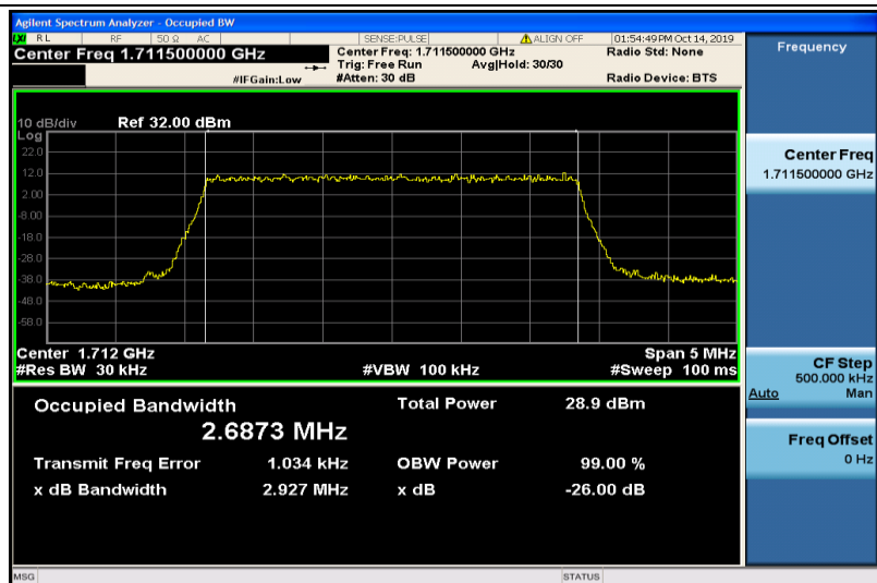
Band4-3MHz-QPSK-19965-15RB#0-2.6873
