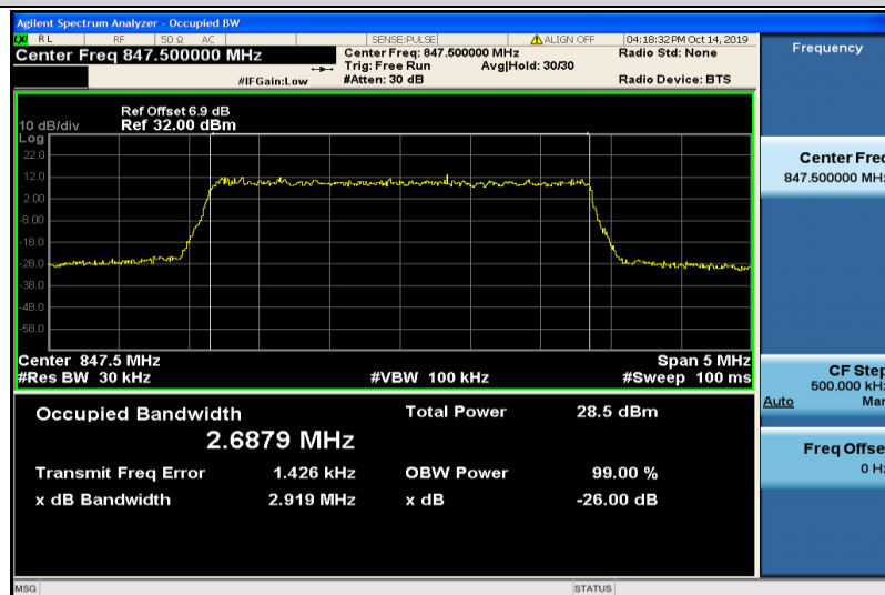
Band5-3MHz-QPSK-20635-15RB#0-2.6879
