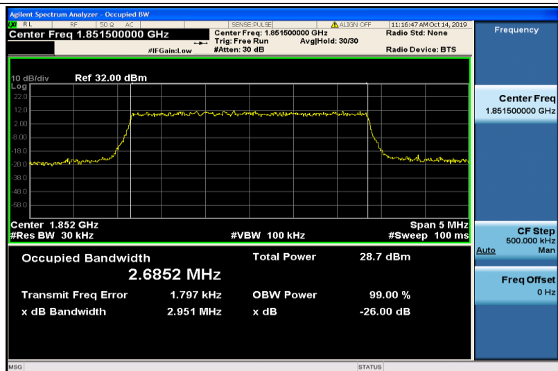
Band2-3MHz-QPSK-18615-15RB#0-2.6852
