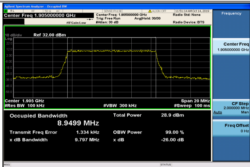
Band2-10MHz-QPSK-19150-50RB#0-8.9499
