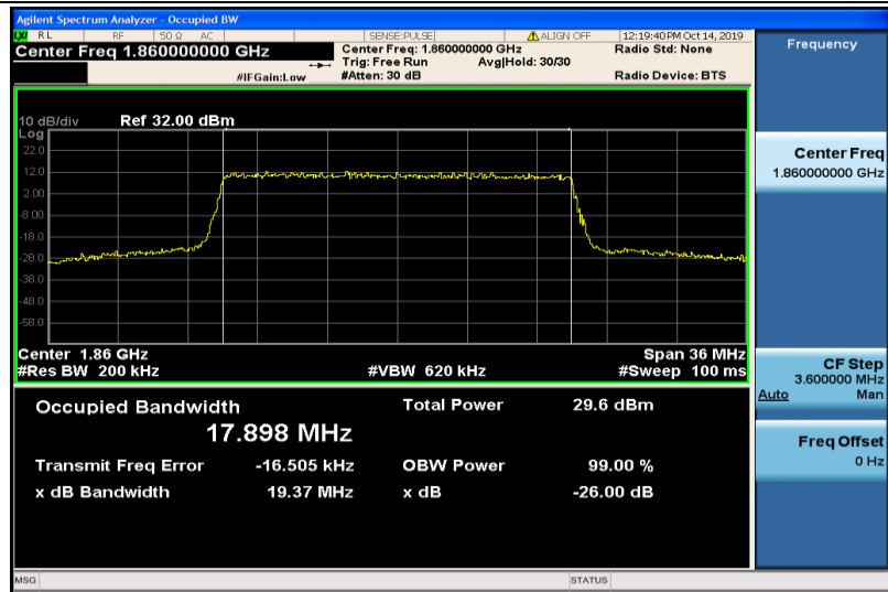
Band2-20MHz-QPSK-18700-100RB#0-17.898
