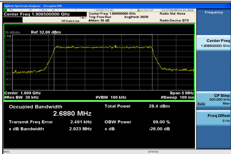
Band2-3MHz-QPSK-19185-15RB#0-2.6880
