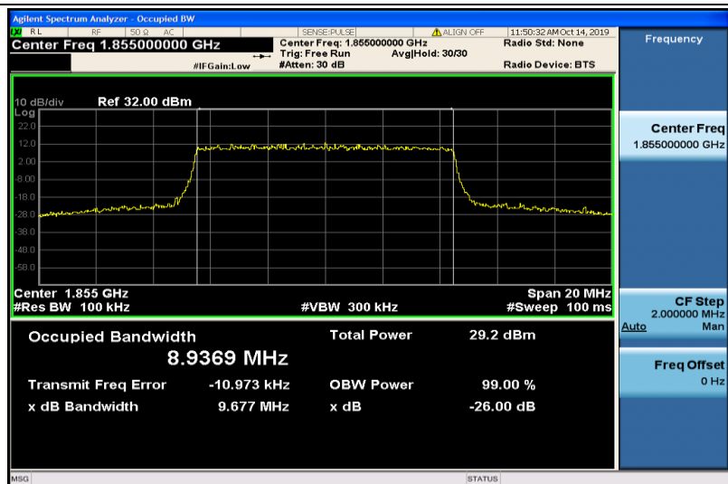
Band2-10MHz-QPSK-18650-50RB#0-8.9369
