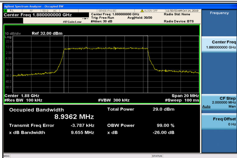
Band2-10MHz-QPSK-18900-50RB#0-8.9362
