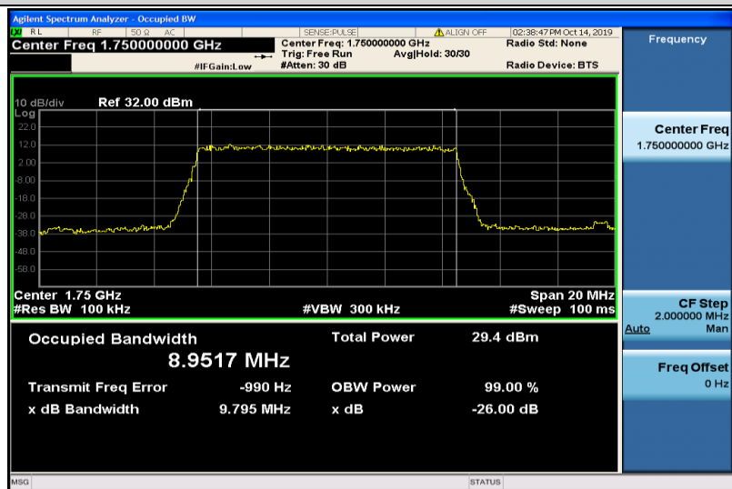
Band4-10MHz-QPSK-20350-50RB#0-8.9517
