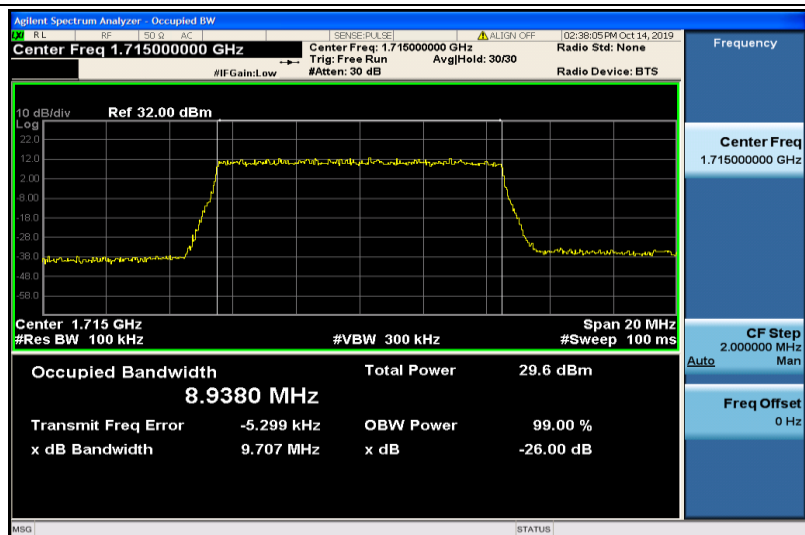
Band4-10MHz-QPSK-20000-50RB#0-8.9380
