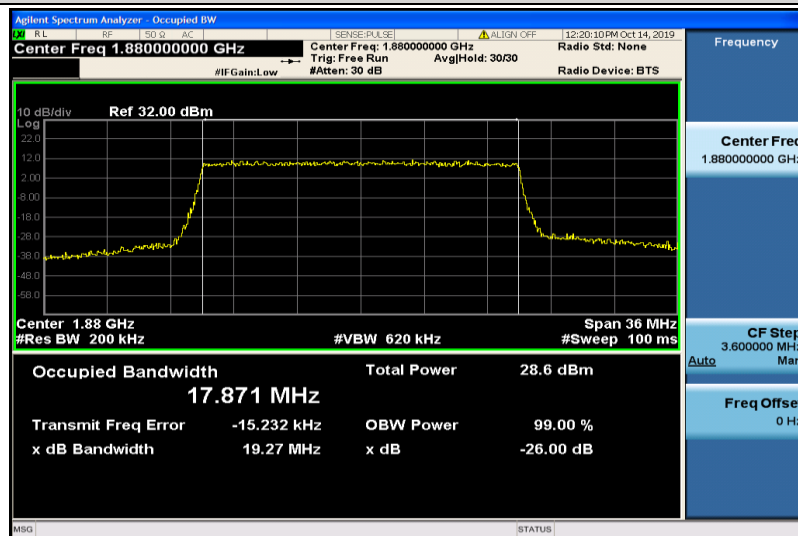
Band2-20MHz-16QAM-18900-100RB#0-17.871
