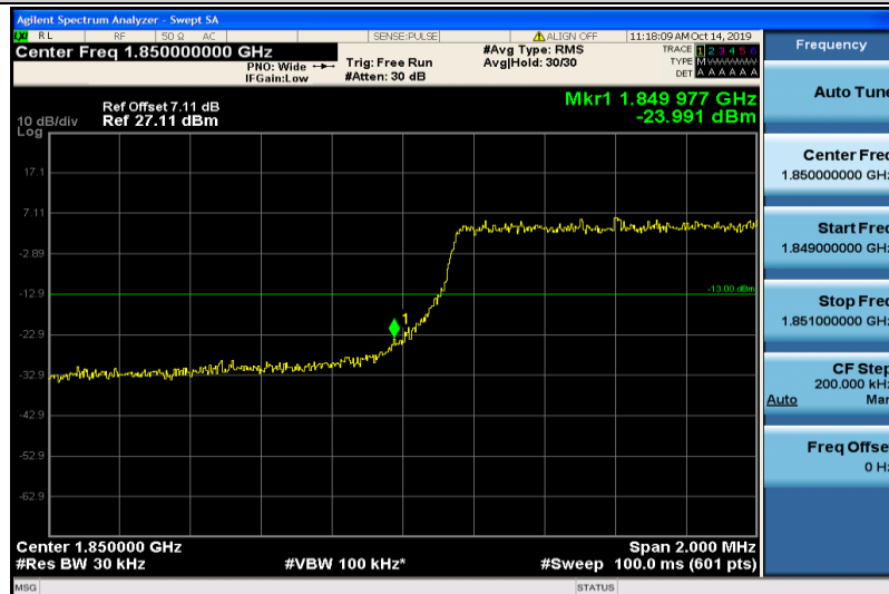
Band2-3MHz-QPSK-18615-15RB#0
