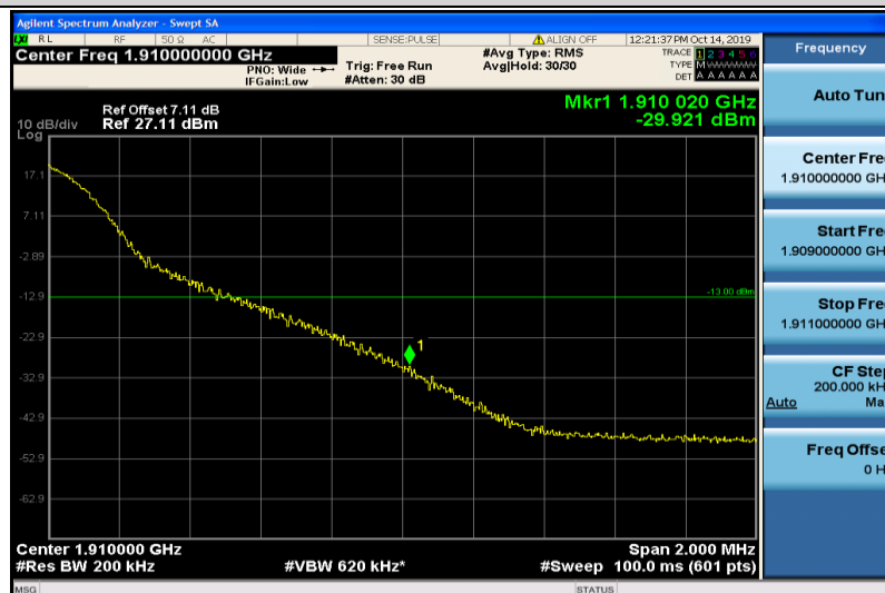
Band2-20MHz-QPSK-19100-1RB#99
