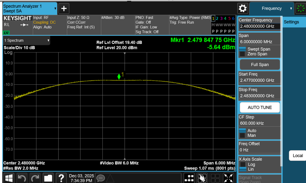
BLE 2M-Ant1-2480-PASS
