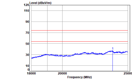
2.4G_SRD_LOW_TX_Horizontal
