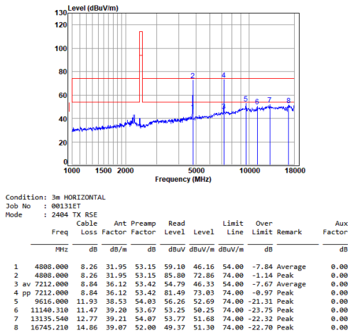
2.4G_SRD_LOW_TX_Horizontal
