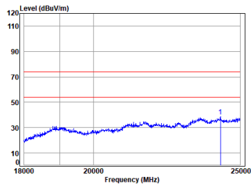
2.4G_SRD_LOW_TX_Horizontal
