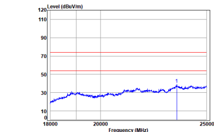
2.4G_SRD_LOW_TX_Horizontal
