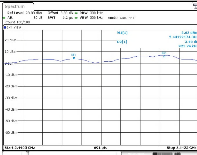
3DH5_Ant1_Hop
