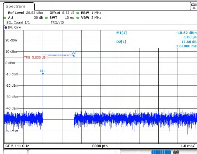
DH5_Ant1_Hop
