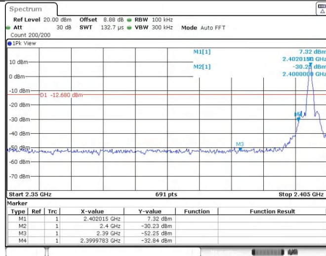
DH5_Ant1_Low_2402
