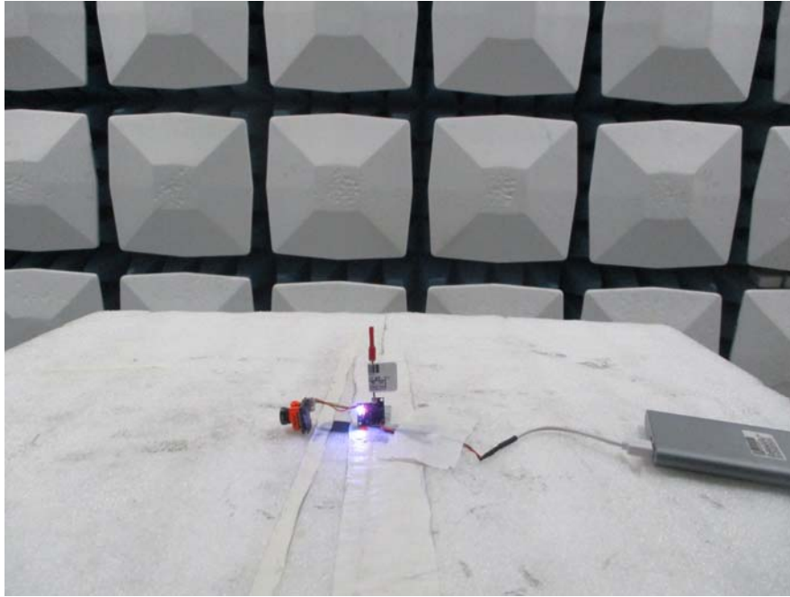
EUT Setup Photo
