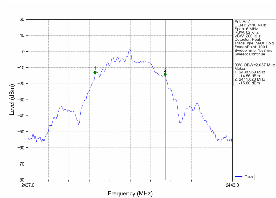
2M_MCH_2440MHz_Ant1_NTNV
