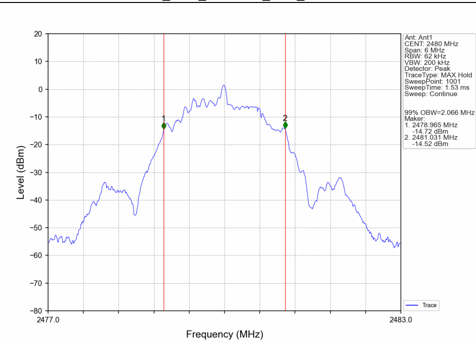
2M_HCH_2480MHz_Ant1_NTNV
