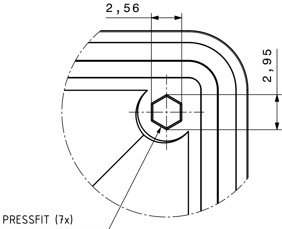
DETAIL C SCALE: 5:1
