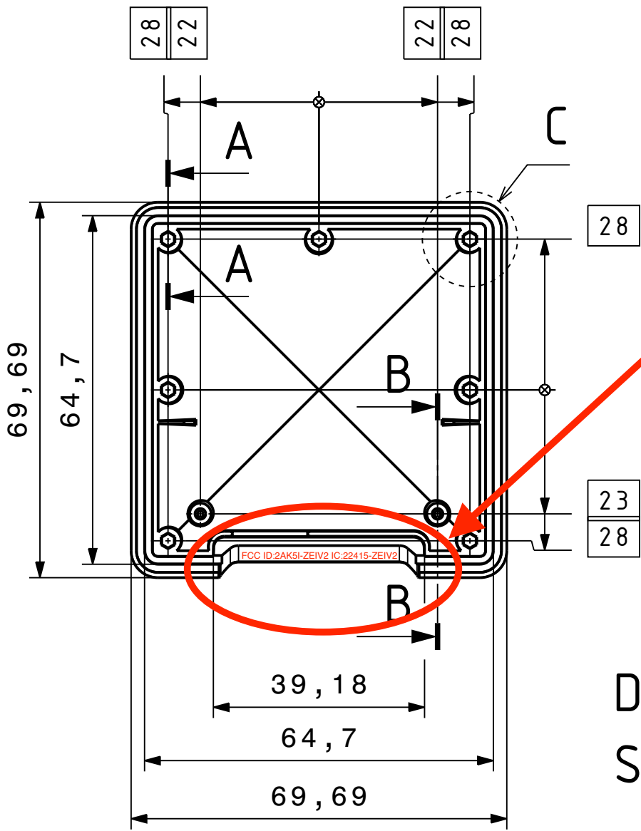
TOP VIEW SCALE: 1:1
