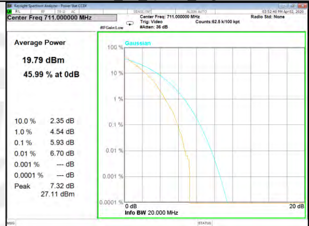
B17_50_Q16_High
