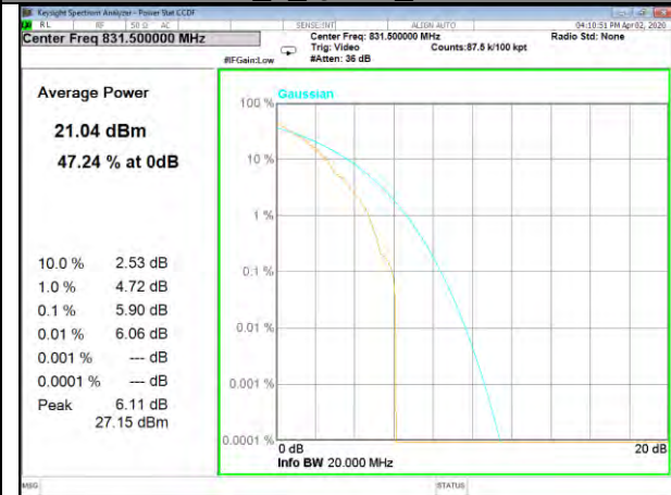
B26_1_Q16_Lower
