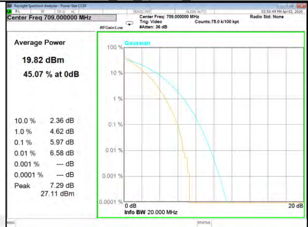
B17_50_Q16_Lower
