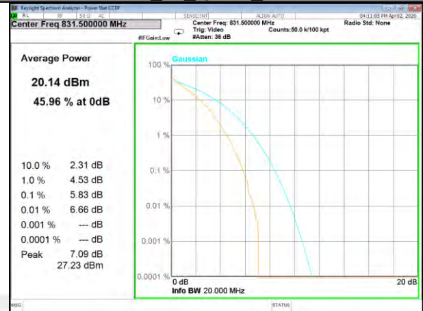
B26_50_Q16_Lower
