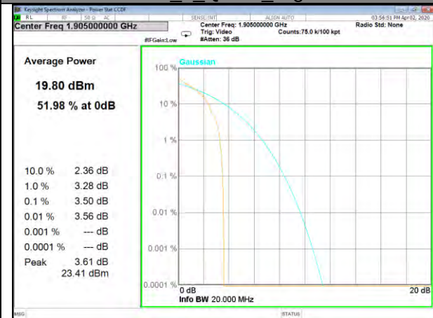
B25_1_Q16_High
