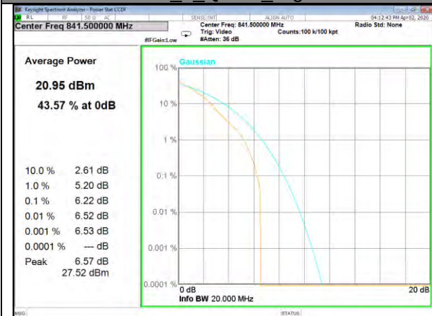
B26_1_Q16_High
