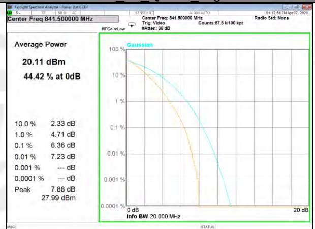
B26_50_Q16_High
