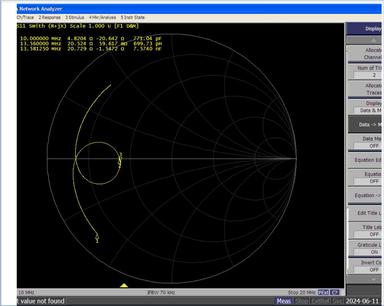
• 阻抗网分图
