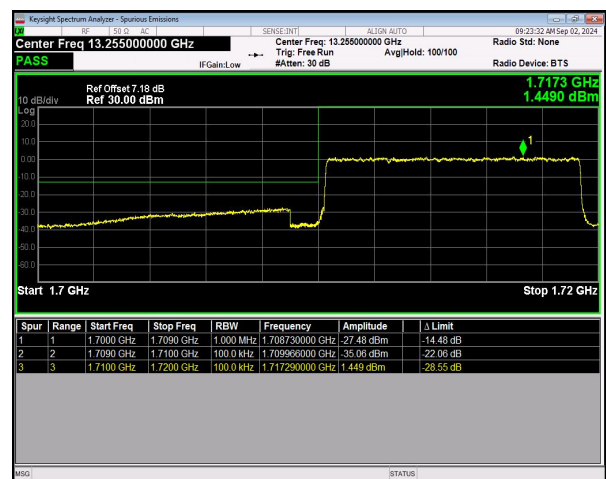
n66 SCS=15kHz DFT_64QAM BW=10MHz LowChannel=343000 RB=50@0 NVNT
