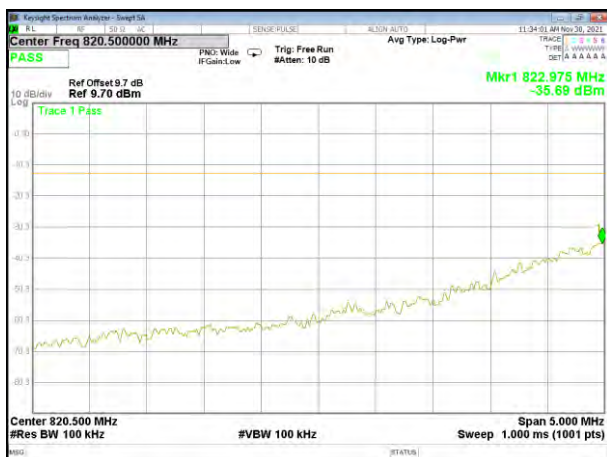
CDMA BC0 Low Band edge
