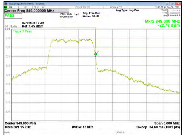
EVDO BC0 High Band edge
