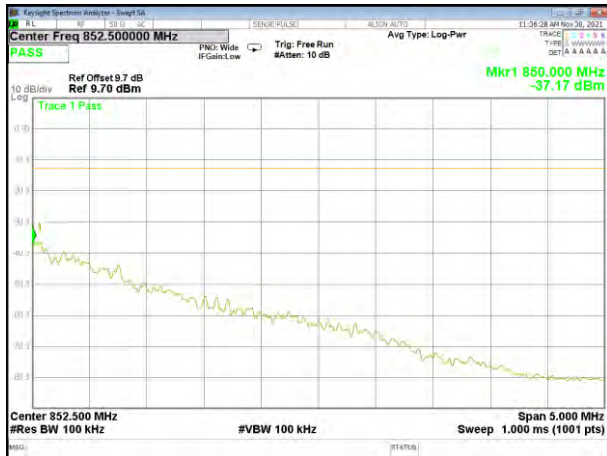
EVDO BC0 High Band edge
