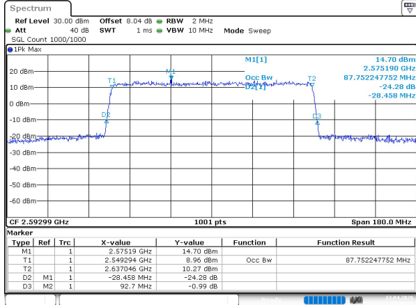
n41 SCS=30kHz CP_16QAM BW=90MHz Channel=518598 RB=245@0
