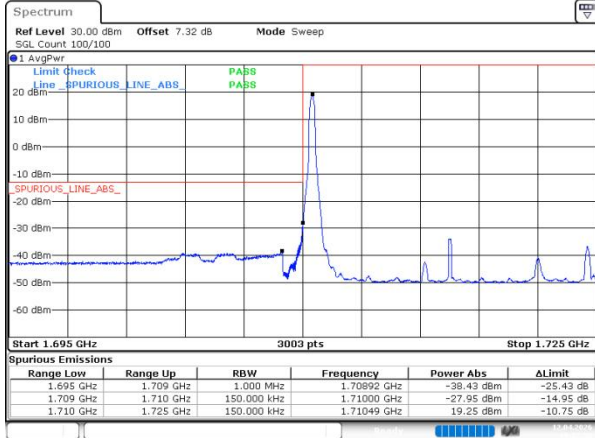
n66 SCS=15kHz DFT_16QAM BW=15MHz LowChannel=343500 RB=1@0
