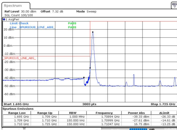
n66 SCS=15kHz DFT_64QAM BW=15MHz LowChannel=343500 RB=1@0
