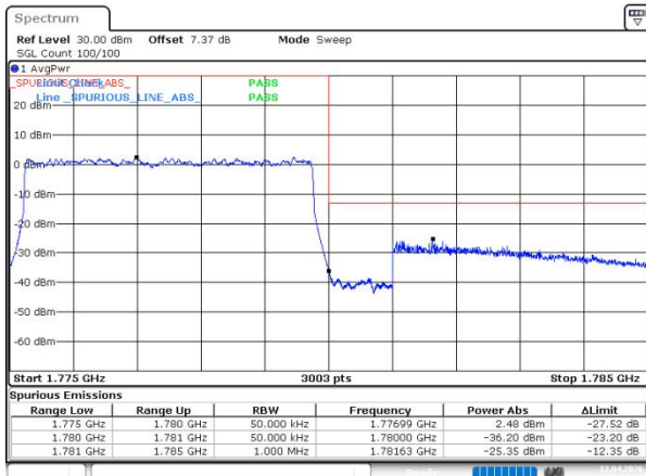
n66 SCS=15kHz DFT_QPSK BW=5MHz HighChannel=355500 RB=25@0
