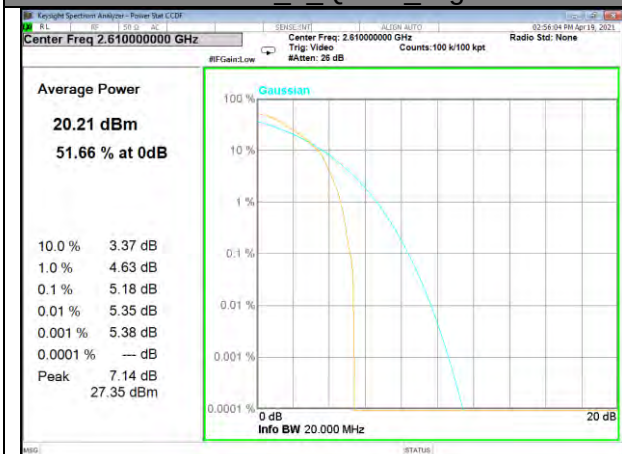
Band 38_1_Q16_High
