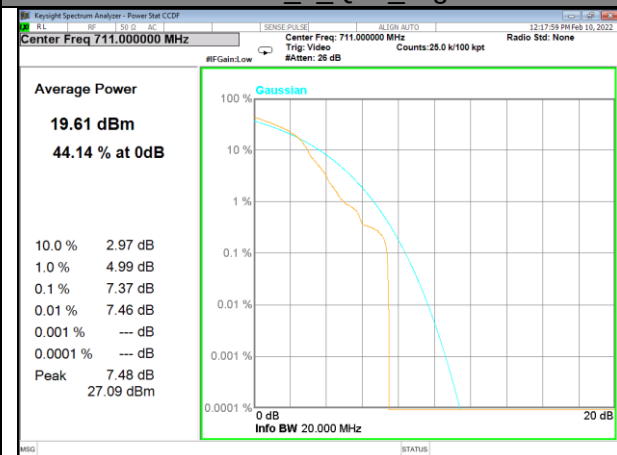
Band 12_1_Q16_High
