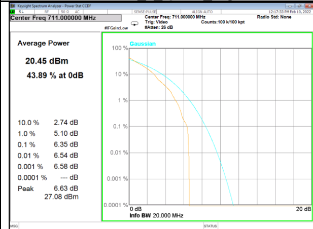
Band 12_1_Q16_High
