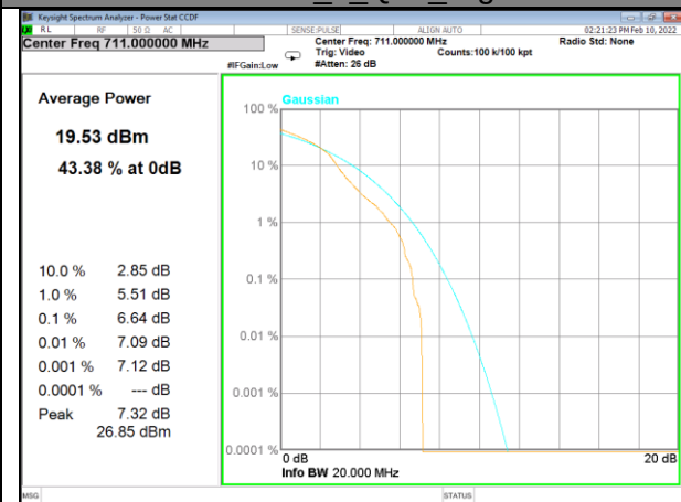
Band 17_1_Q16_High
