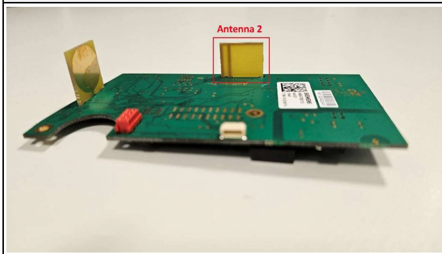
Antenna 2 - Bottom
