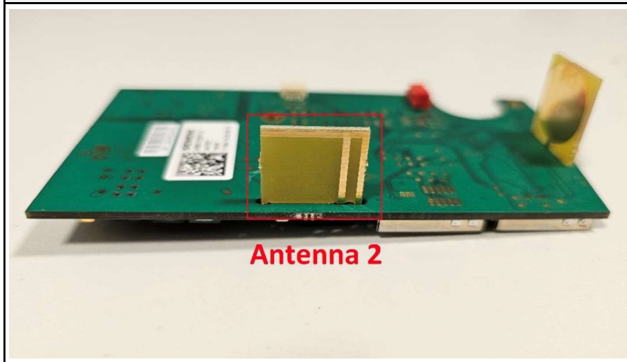
Antenna 2 - Top
