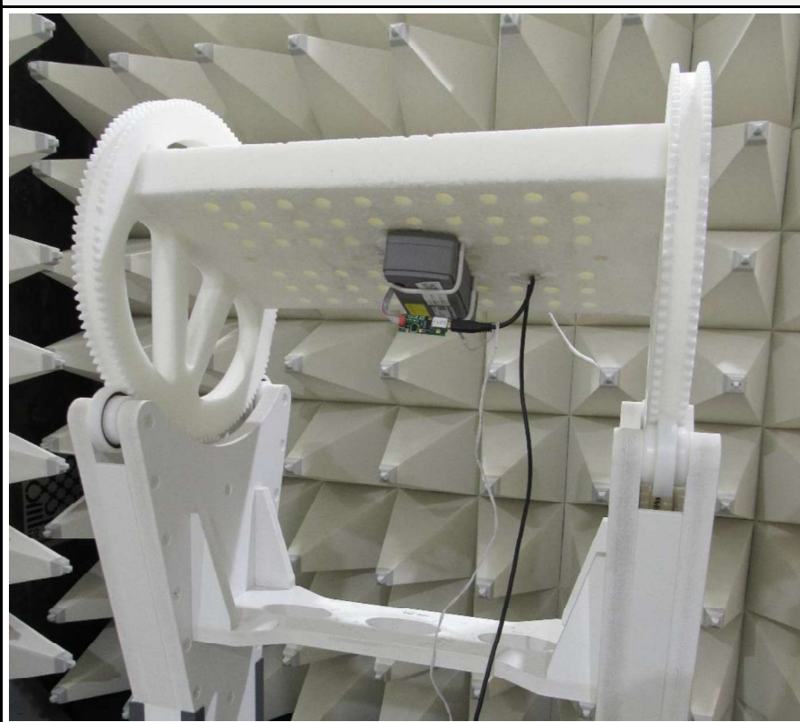
Setup EUT
