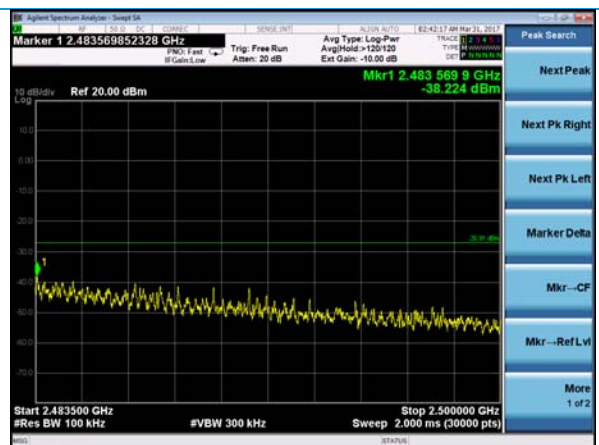
54 Mbps – Upper Band Edge
