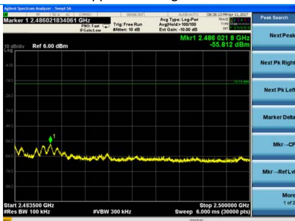
BLE – Upper Band Edge
