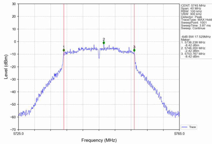
802.11n(HT20) LCH 5745MHz_Ant1_NTNV
