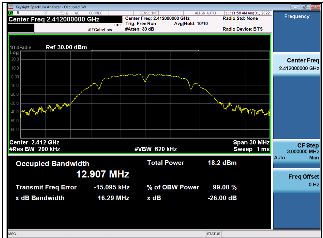
Test_Graph_802.11b_ANT3_2412_1Mbps_OBW
