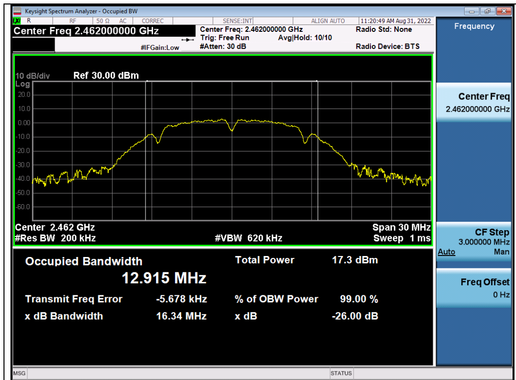
Test_Graph_802.11b_ANT3_2462_1Mbps_OBW
