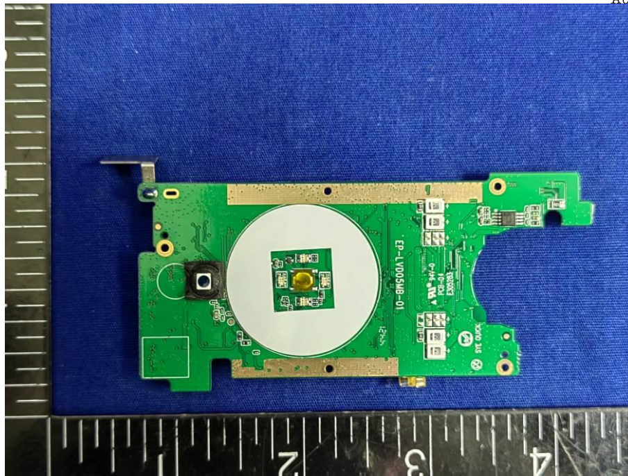
RFID Antenna
