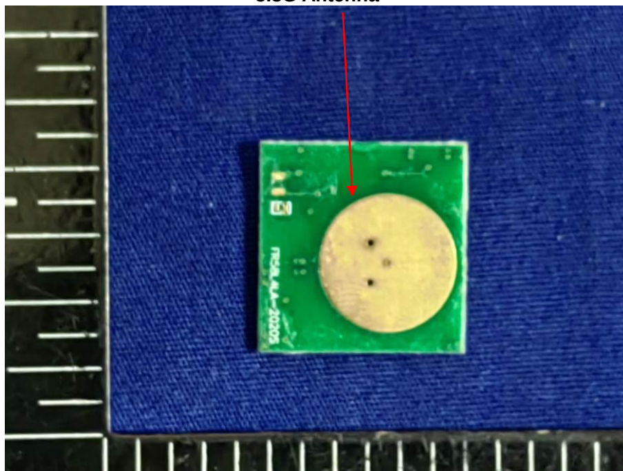
5.8G Antenna
