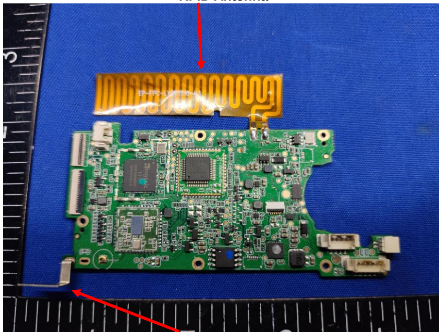
BLE & WiFi antenna
