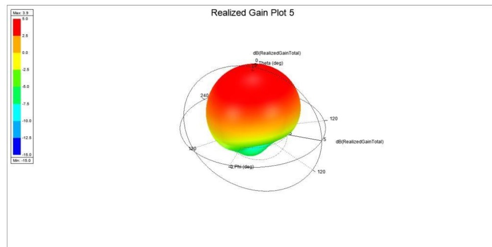
图八 3D方向图 5.826 GHz
