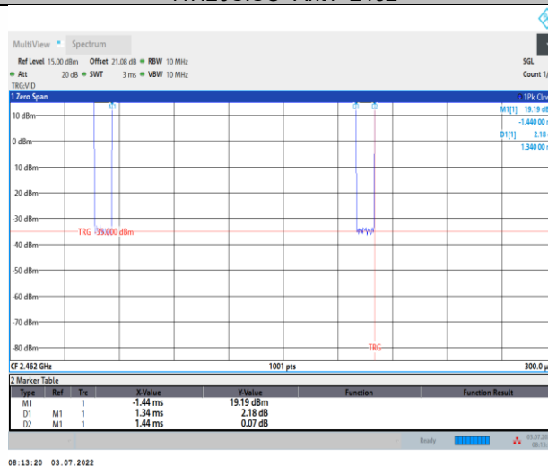
11N20SISO_Ant1_2462
