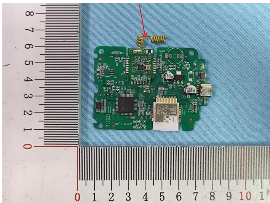
915MHz-ANT
