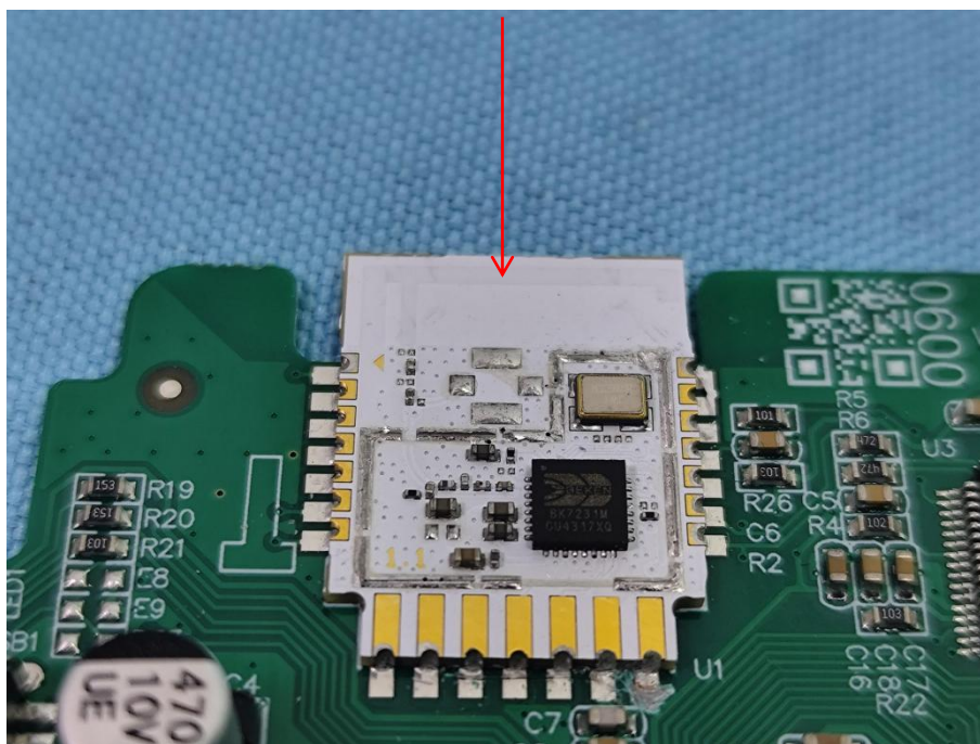
BLE&WiFi-ANT
