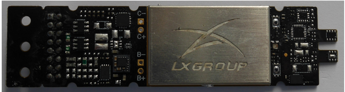
PCB bottom
