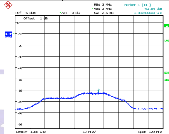
Uplink, 1850-1910MHz
