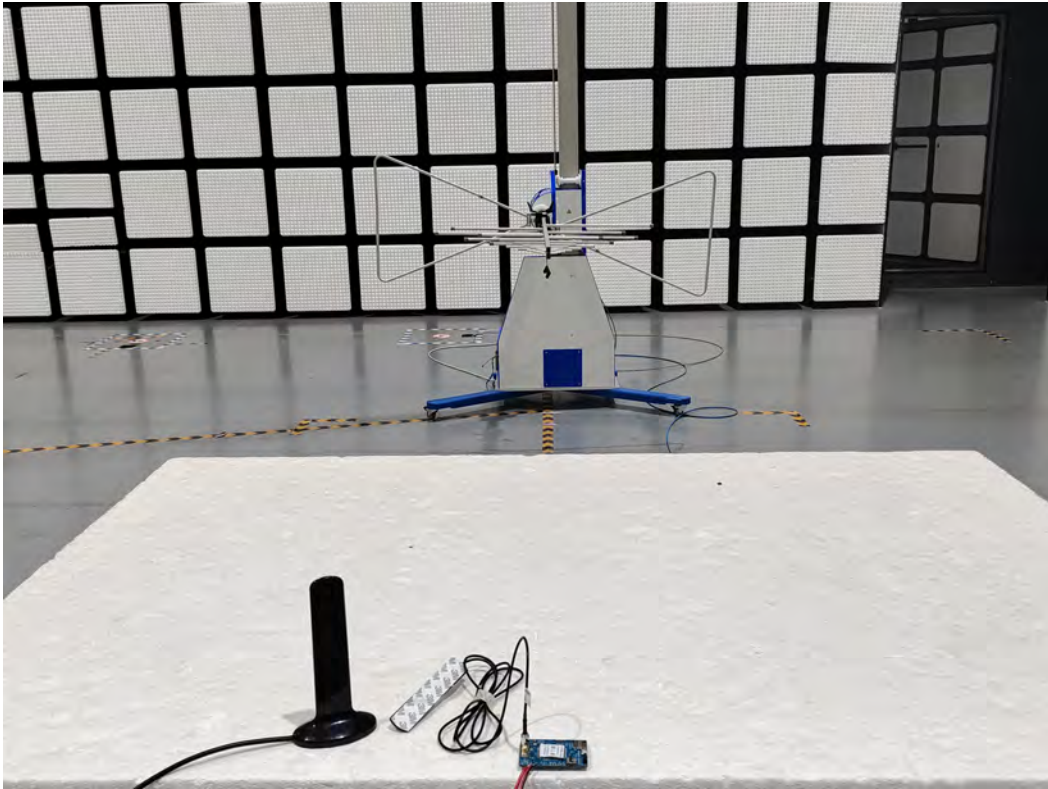
Pic1.RSE(30MHz-1GHz)
