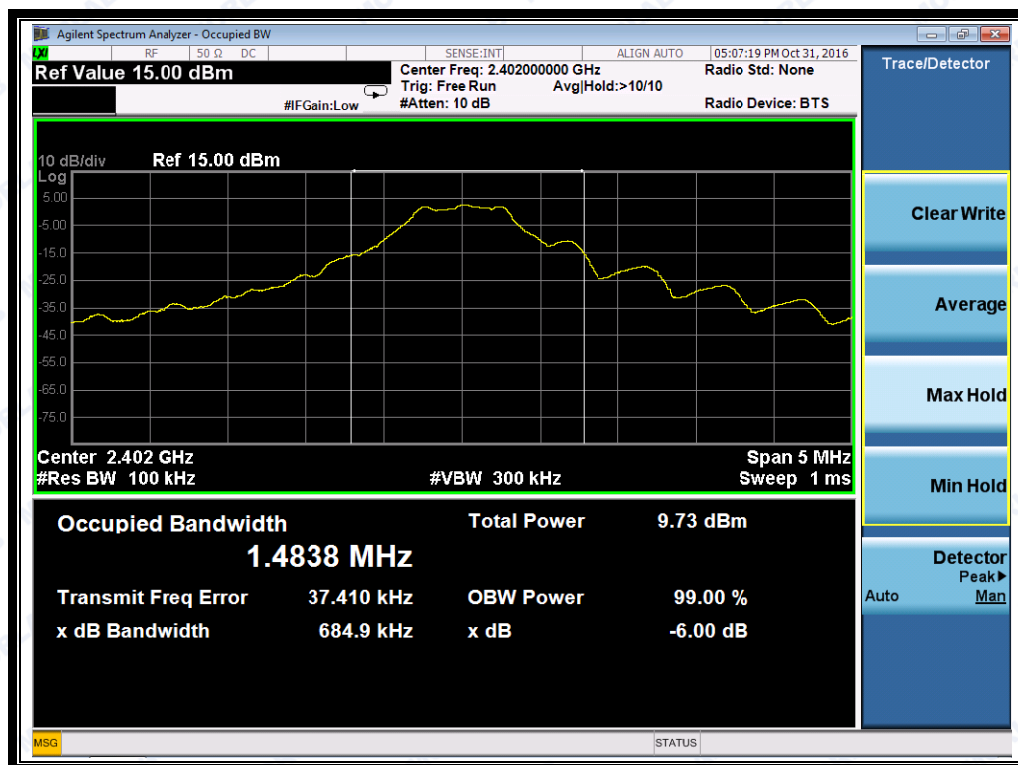
(Plot A: Channel 3: 2402MHz)
