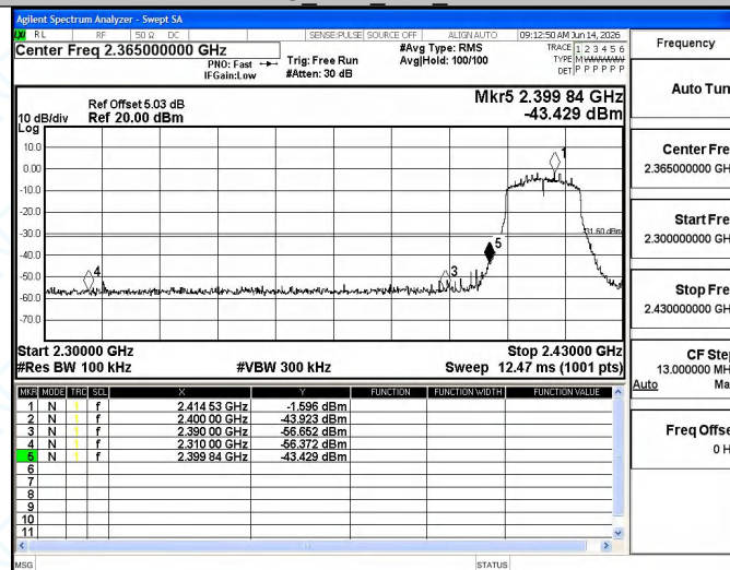
11G_Ant1_Low_2412
