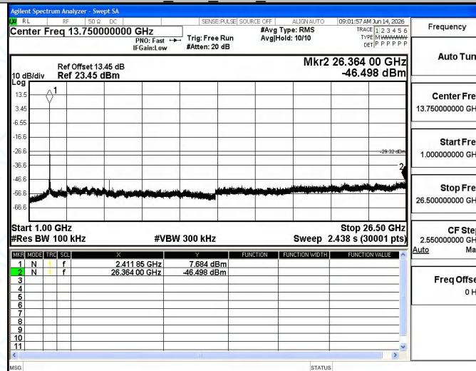
11B_Ant1_2412_1000~26500
