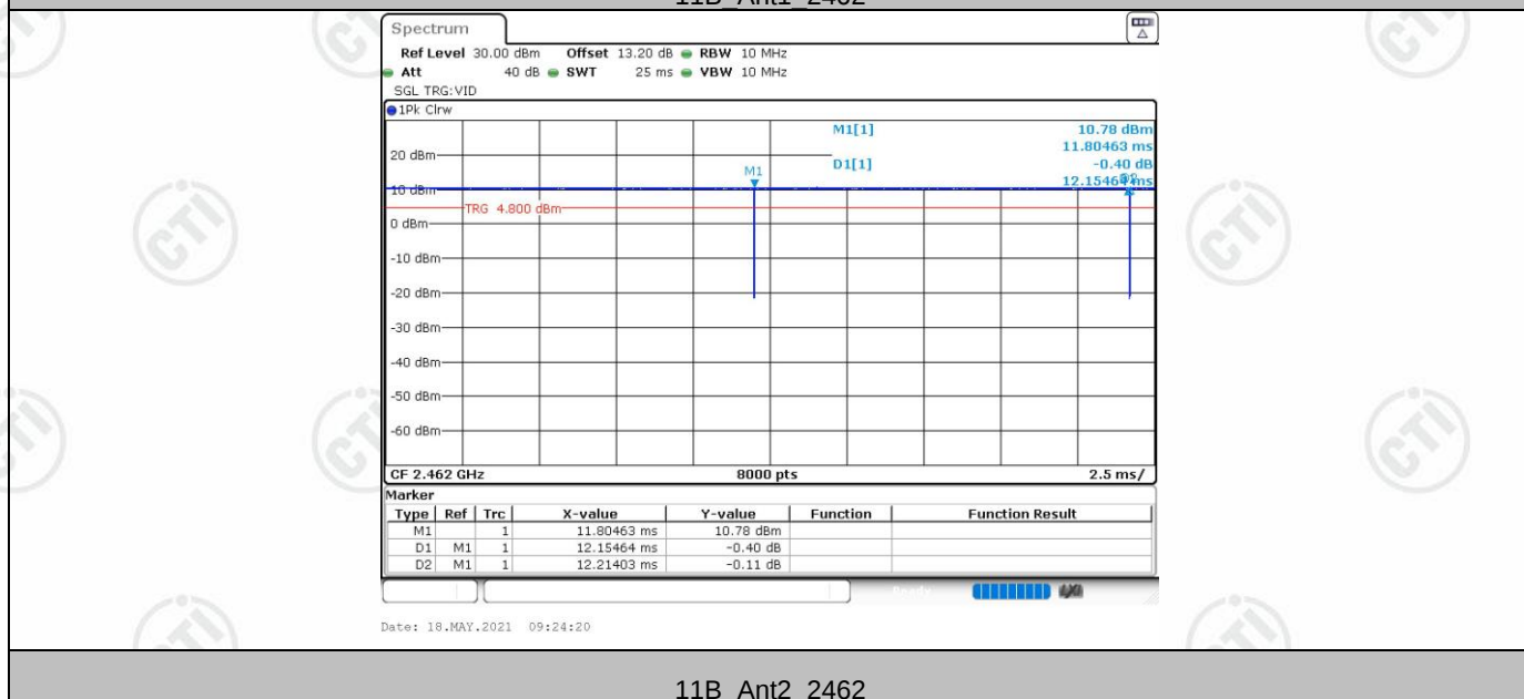
11B Ant1 2462
