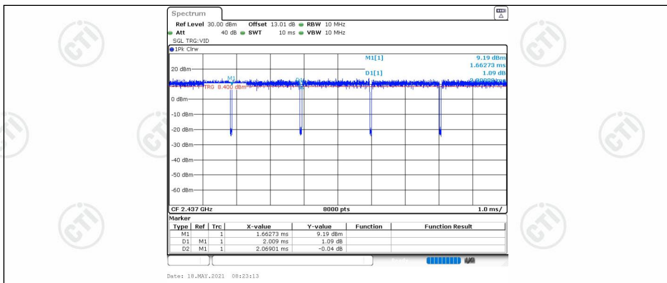
11G Ant1 2437
