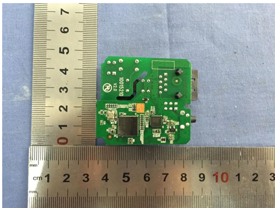
P200 Module(PLC)
