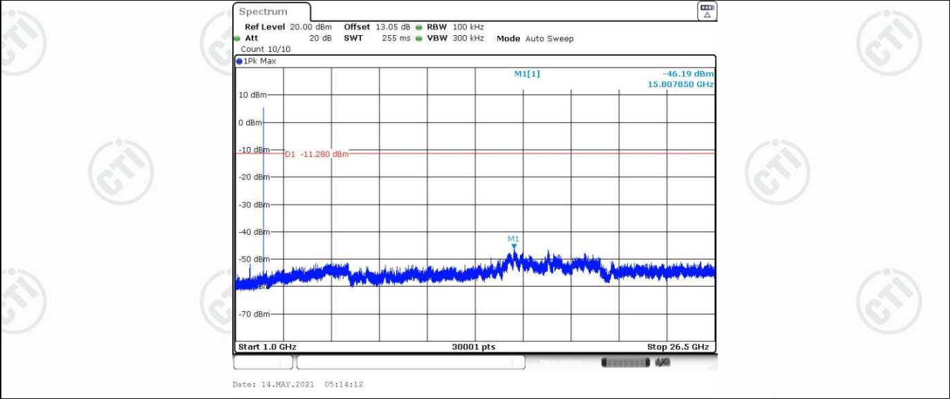
OTHER Ant1 2475 1000~26500
