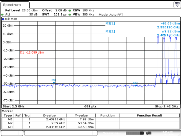
OTHER_Ant1_Low_hop
