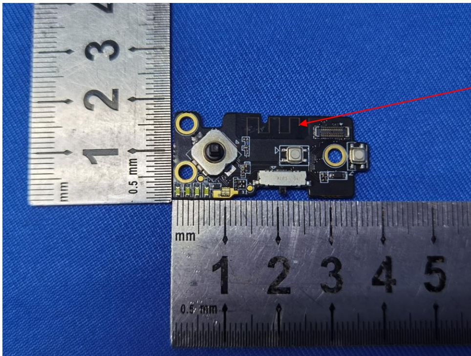
BLE antenna
