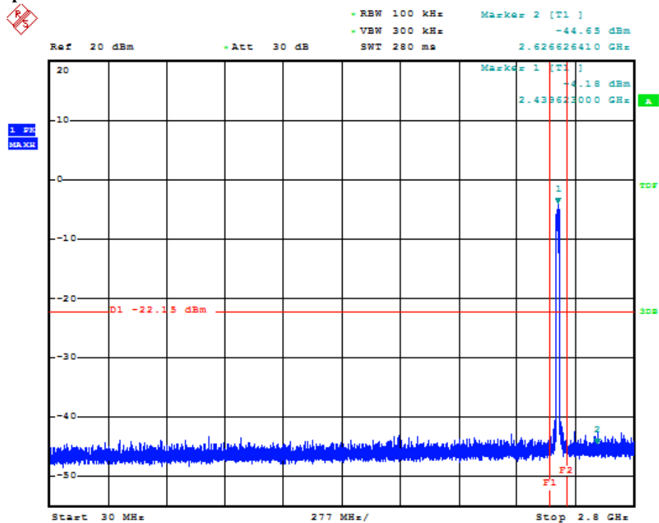
20dBc-30MHz-2.8GHz-Ch6-nMode-MCS0
