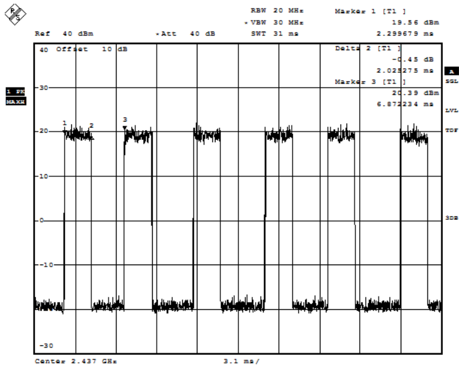
DC_CH6_6Mbit
