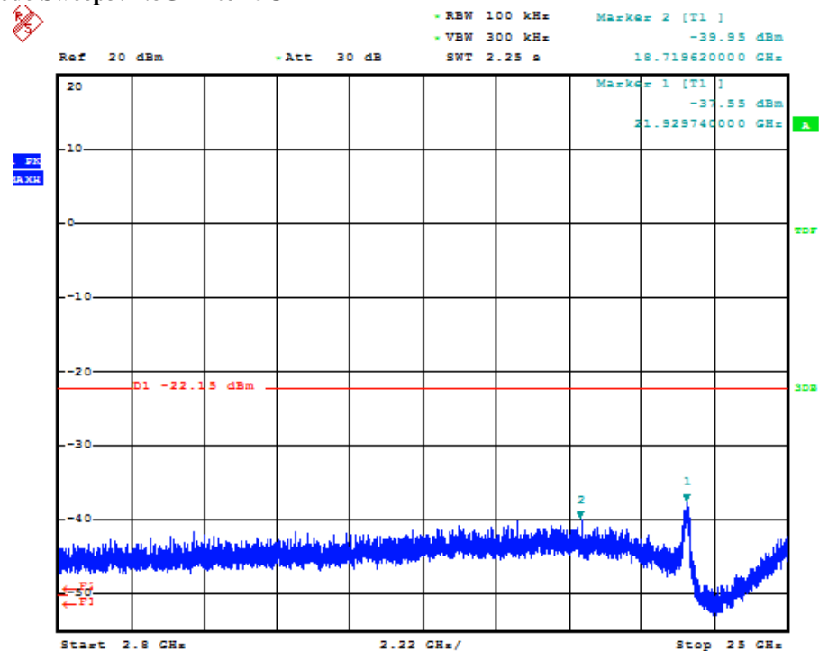
20dBc-2.8GHz-25GHz-Ch6-nMode-MCS0
