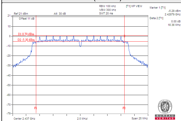
802.11n (VHT20)
