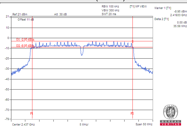
802.11n (VHT40)
