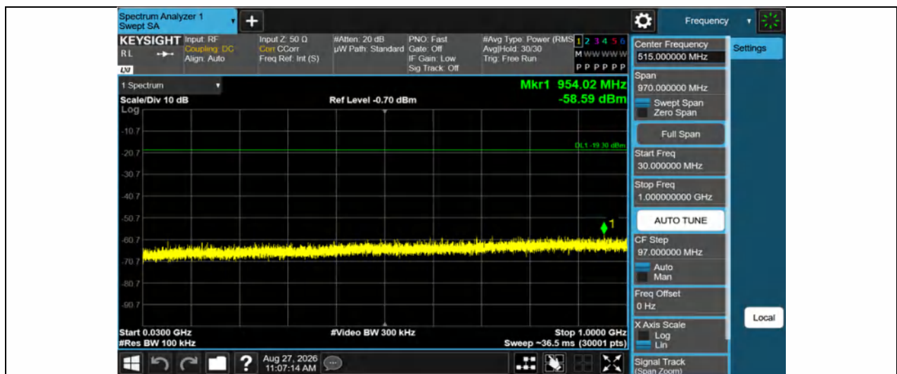
11G-Ant1-2412-30~1000-PASS
