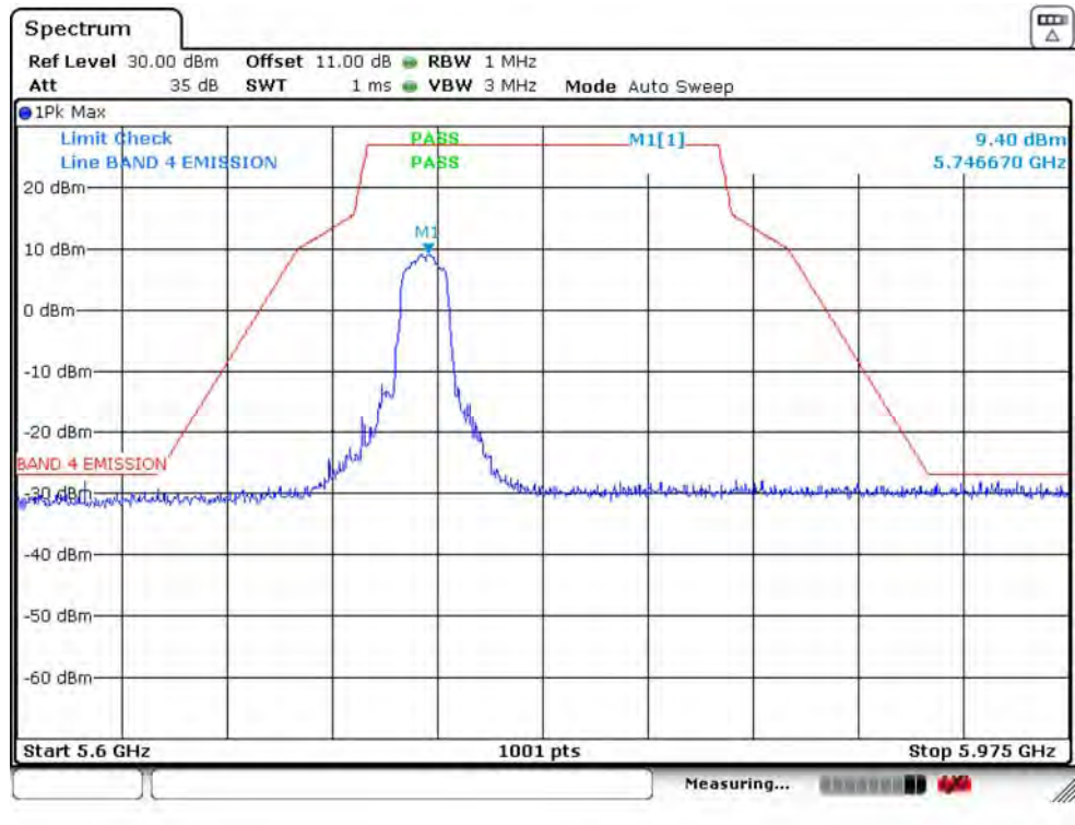
IEEE 802.11a 5745 MHz
