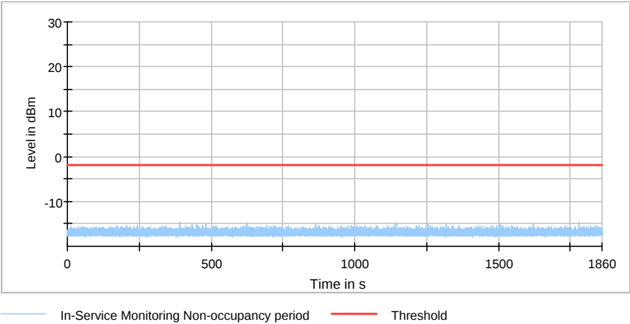
802.11a 5260MHz
