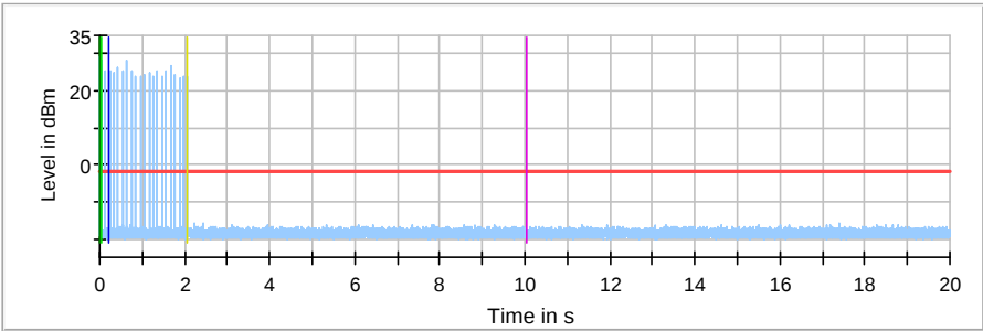
802.11a 5260MHz
