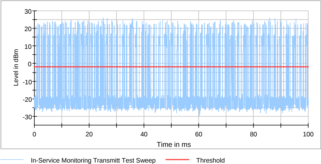
802.11a 5260MHz
